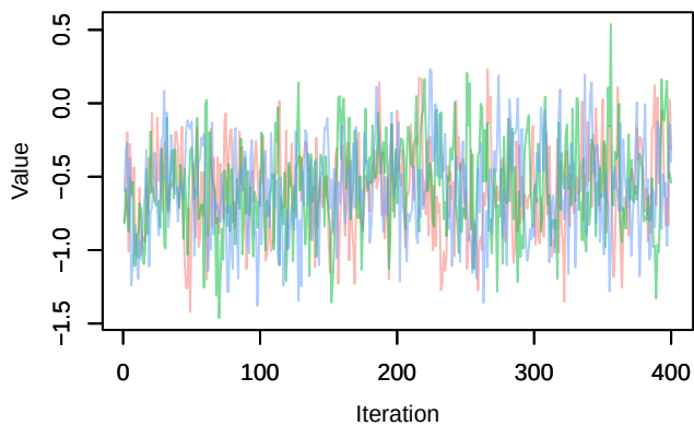
Trace – beta1[5]
