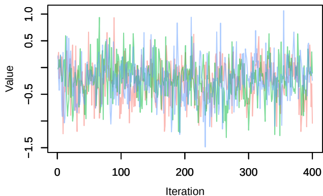
Trace – beta1[5]
