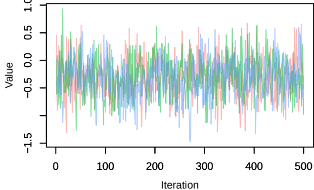
Trace – beta1[5]
