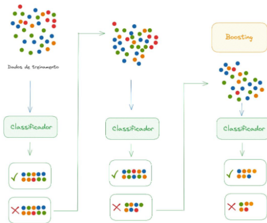
Figura 14 – Estrutura do Boosting
