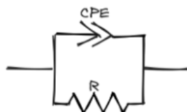
Figura 8 – Representação do circuito RC.
