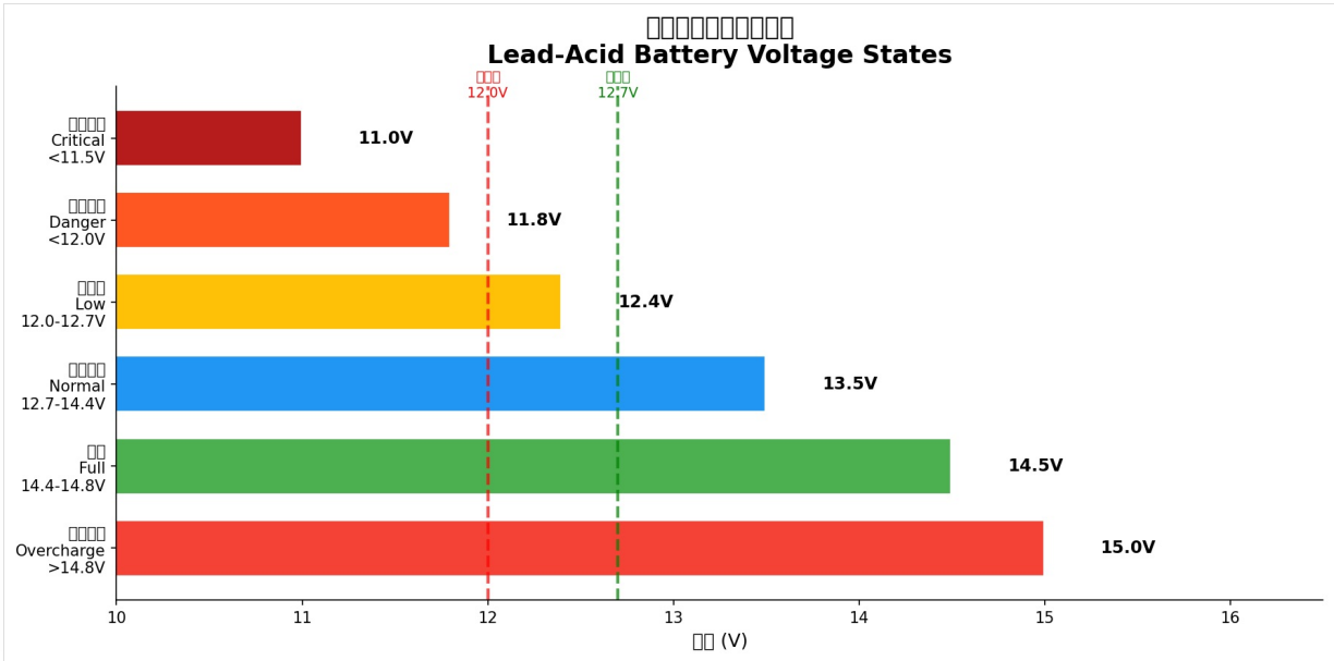
圖4-2：鉛酸蓄電池電壓狀態表
