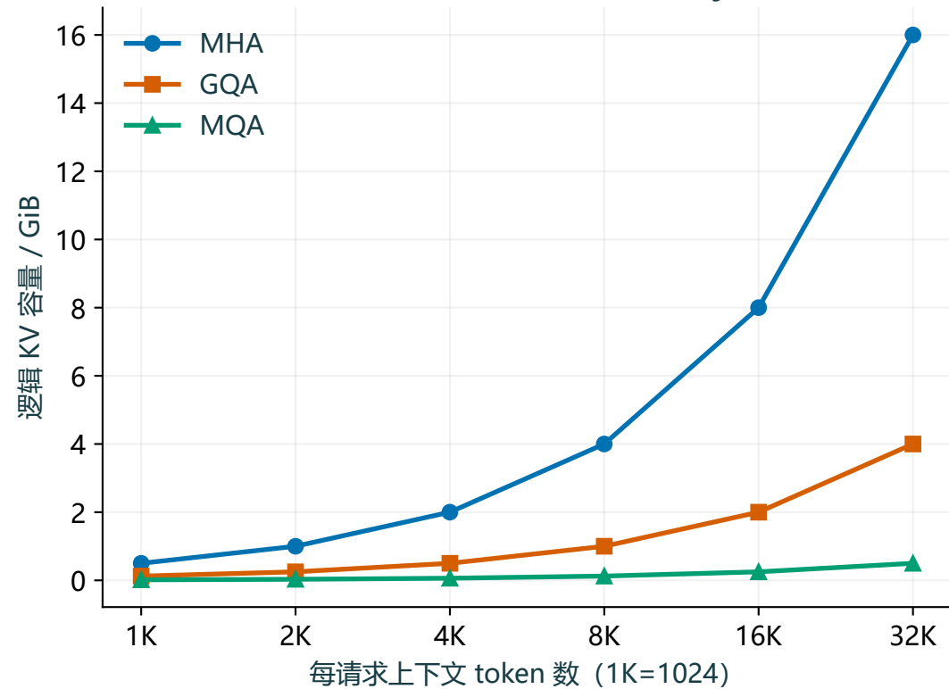
单请求: L=32, d=128, s=2 bytes
