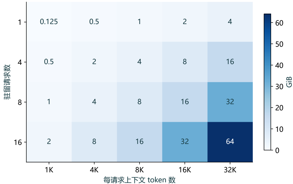
GQA • Hkv=8: 并发使容量相乘
