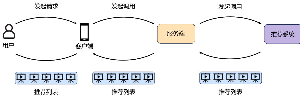
图 1.3: 一次完整的用户推荐请求流程。
