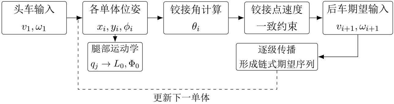
图 2: 第 2 章链式系统运动学建模框图
