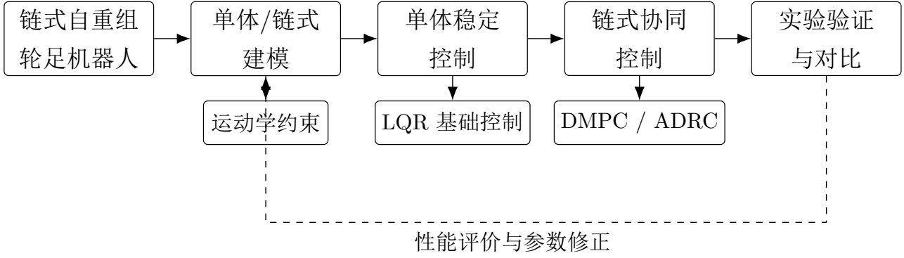
图 1: 第 1 章研究内容与控制方案总体关系框图
