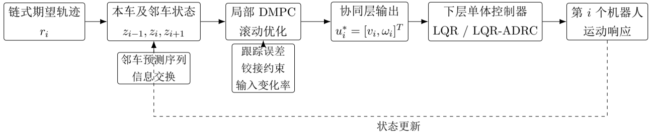
图 4: 第 4 章分层 DMPC 协同控制框图
