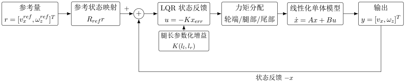
图 3: 第 3 章单体 LQR 基础控制闭环框图
