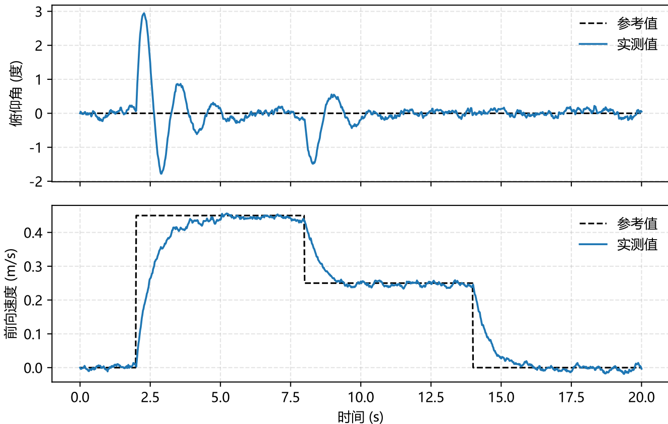
单体 LQR 控制响应
