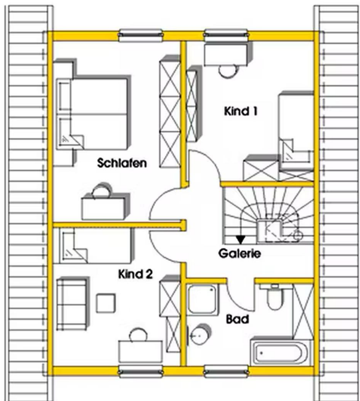
Dachgeschoss
