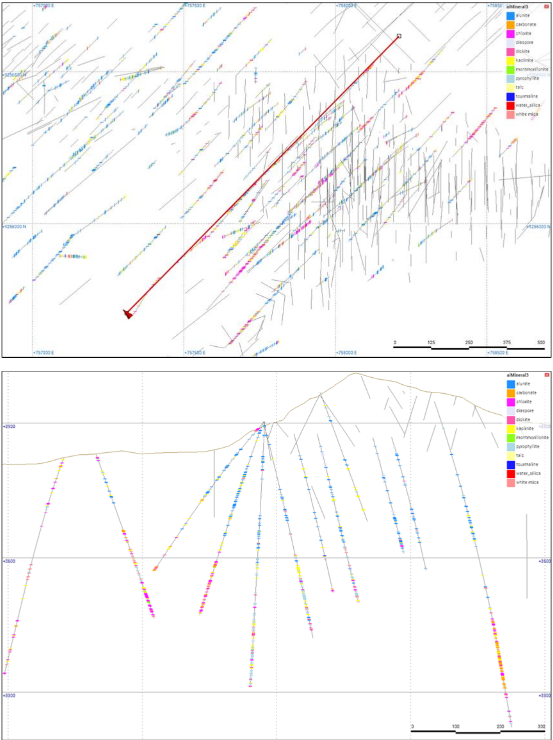
Planta y Sección del tercer mineral más abundante de la zona del SWIR por muestra
