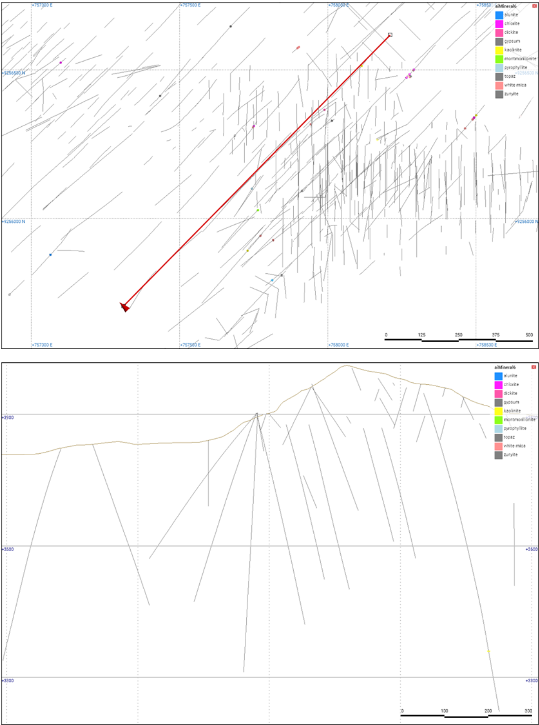
Planta y Sección del sexto mineral más abundante de la zona del SWIR por muestra
