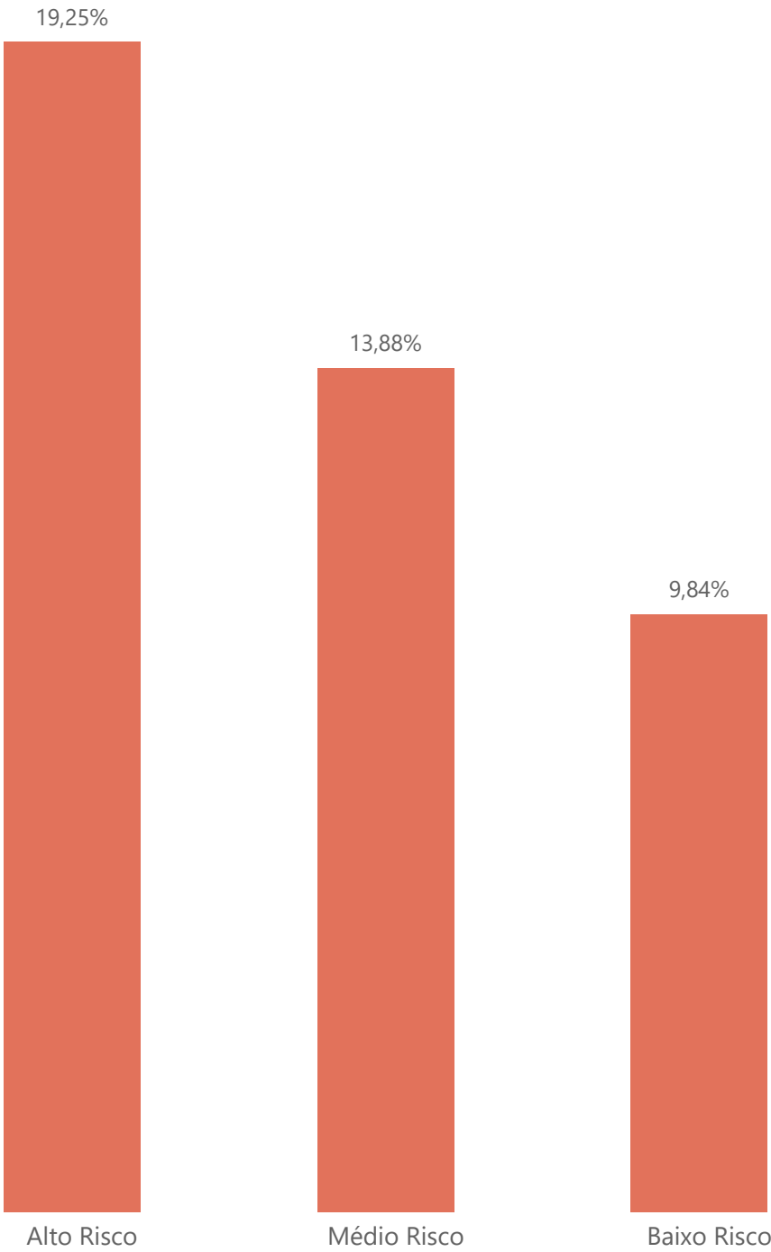
Taxa de Inadimplência por Faixa de Score
