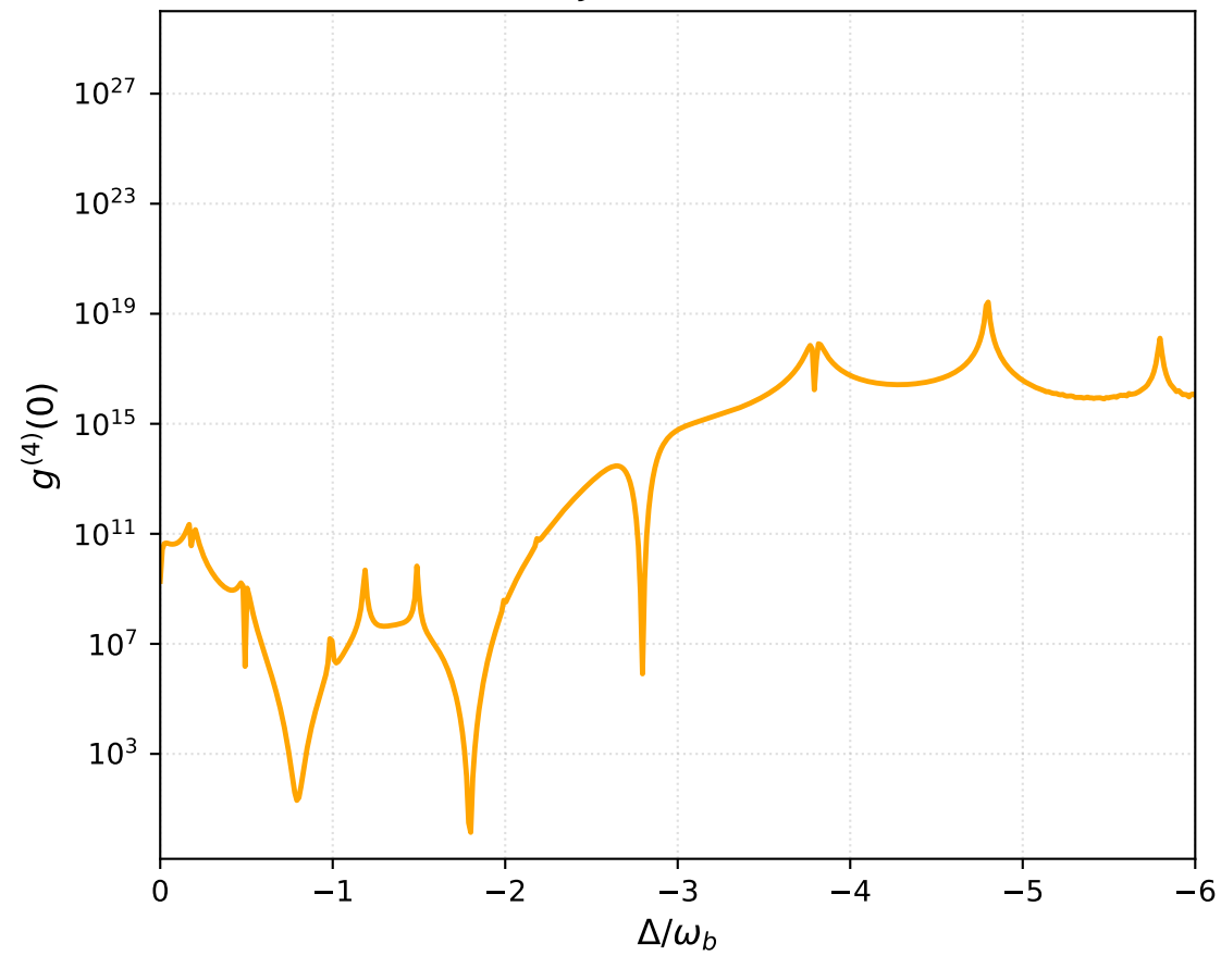
J/\omega b = 0.8
