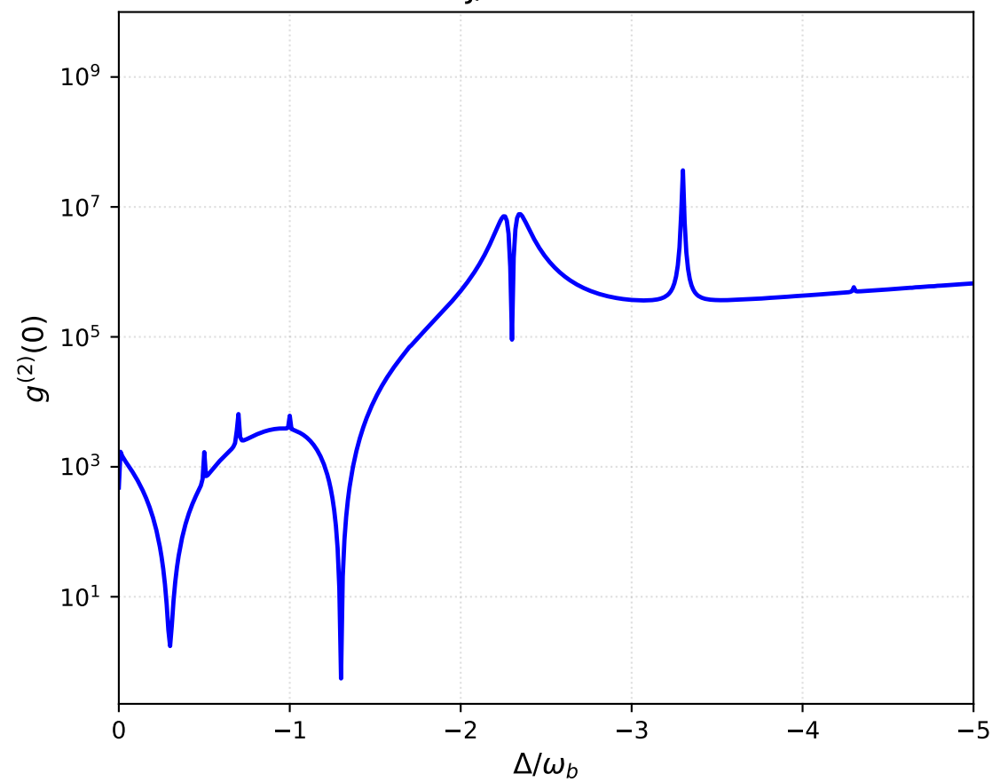
J/\omega b = 0.8
