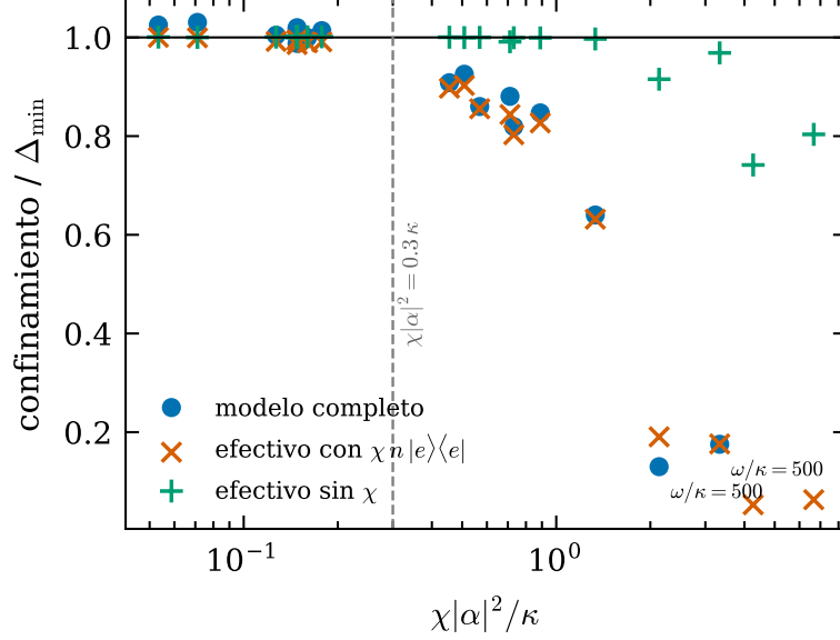
Figura 4: Confinamiento del modelo completo relativo al del modelo mínimo frente a \chi|\alpha|^2/\kappa . Círculos: modelo completo. Cruces: efectivo con \chi n|e\rangle\langle e| . Signos +: efectivo sin \chi . La línea discontinua marca \chi|\alpha|^2 = 0.3\kappa . Los puntos con \omega/\kappa = 500 están rotulados; con \omega/\kappa = 1000 el gato no se estabiliza y no hay punto del modelo completo.
