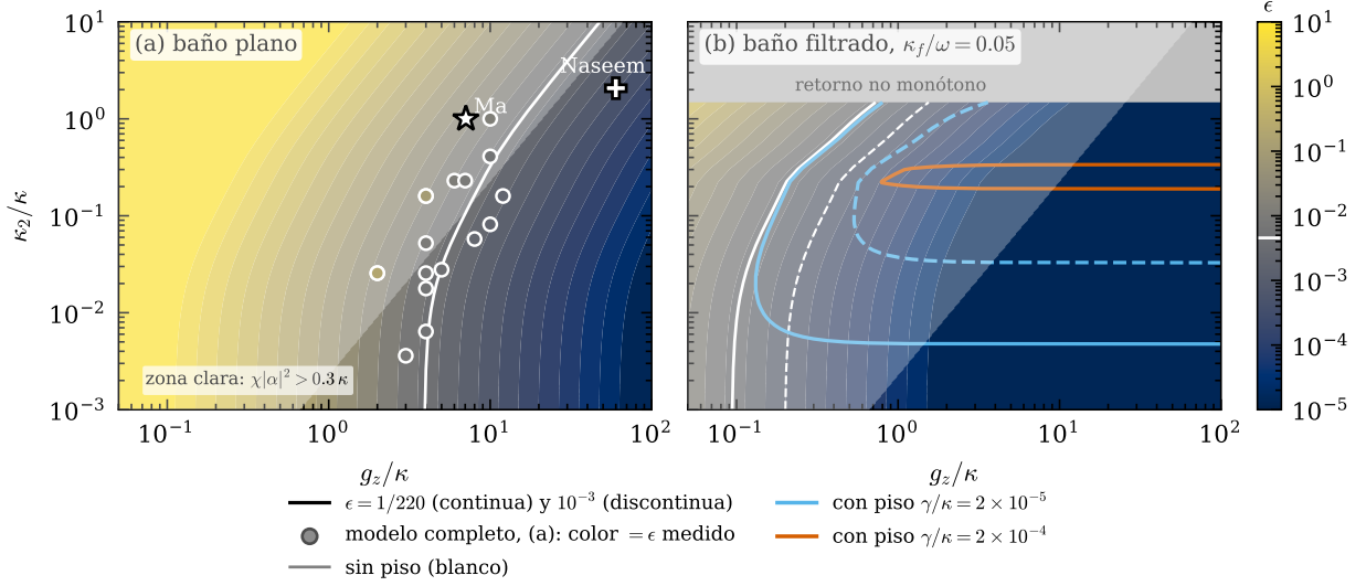
Figura 5: Mapa de diseño: \epsilon = \kappa_1/\kappa_2^{\text{eff}} para |\alpha|^2 = 4 y \omega/\kappa = 200 , en el plano (g_z/\kappa, \kappa_2/\kappa) , con el costo del filtro en confinamiento incluido. (a) Baño plano; círculos: 15 puntos del modelo completo ( N = 22 ), coloreados con el \epsilon medido; estrella: Ma; cruz: Naseem (su \omega/\kappa = 1000 hace que la zona clara, calculada con \omega/\kappa = 200 , no le aplique). (b) Baño filtrado con \kappa_f/\omega = 0.05 ; en gris, \kappa_2/\kappa > 1.5 , donde el retorno de P_c no es monótono y la tasa no está definida. Contornos blancos: sin piso intrínseco. Contornos de color: con piso \gamma/\kappa = 2 \times 10^{-5} (celeste) y 2 \times 10^{-4} (naranja). La zona clara es \chi|\alpha|^2 > 0.3\kappa .
