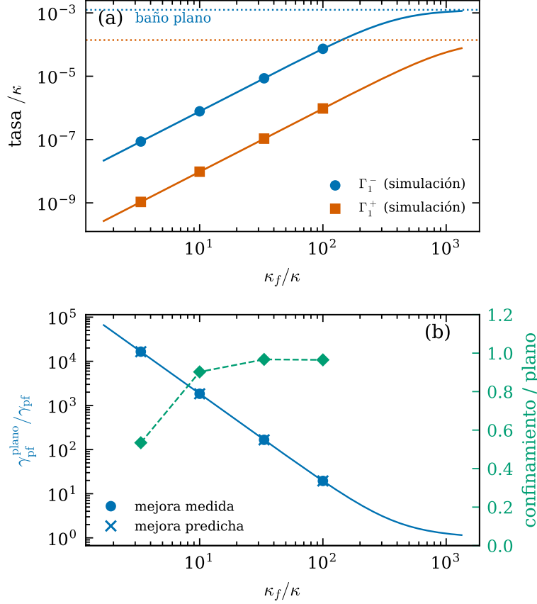
Figura 3: Baño filtrado ( \omega/\kappa = 200 , |\alpha|^2 = 2 ). (a) Tasas de un fonón, \Gamma_1^- y \Gamma_1^+ , normalizadas a \kappa , frente a \kappa_f/\kappa : puntos de la simulación y curvas de la Ec. (62); líneas punteadas: baño plano. (b) Mejora de \gamma_{pf} respecto del baño plano, medida y predicha con la Ec. (54) (eje izquierdo), y tasa de confinamiento relativa al plano (eje derecho).
