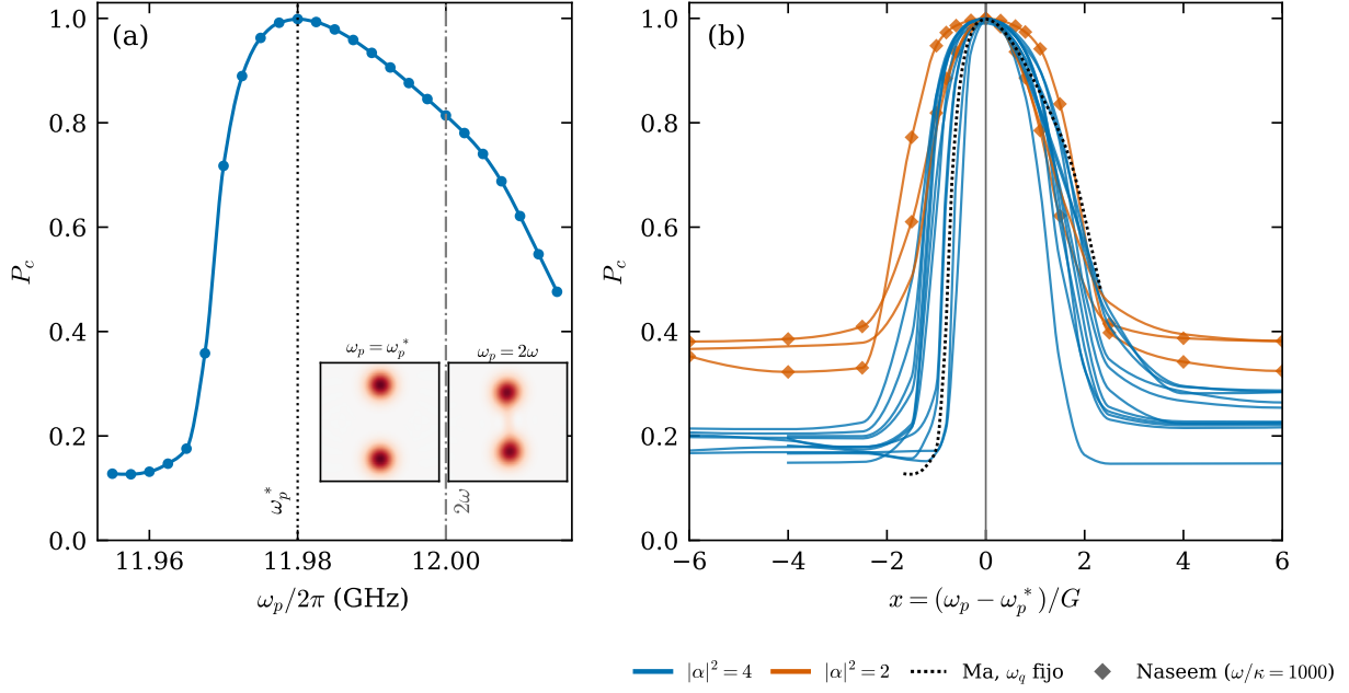
Figura 1: Resonancia vestida. (a) P_c frente a \omega_p en el modelo completo de Ma et al. ( N = 22 , código polarónico fijo). La línea punteada es \omega_p^* = 2(\omega - 4g_x^2/3\omega) = 11.980 y la de trazo y punto es 2\omega . Los recuadros muestran la función de Wigner del oscilador (qubit trazado) en cada punto: dos lóbulos en \pm 2i con el drive en \omega_p^* (gato) y lóbulos con peso fuera del código con \omega_p = 2\omega (sin gato). El código sin desplazar da una curva indistinguible a esta escala (véase el texto). (b) P_c frente a x = (\omega_p - \omega_p^*)/G para 157 estados estacionarios de plataformas distintas: azul, |\alpha|^2 = 4 ; naranja, |\alpha|^2 = 2 ; rombos, parámetros de Naseem ( \omega/\kappa = 1000 ); línea negra punteada, Ma con \omega_q fijo. Todas las curvas centran el pico en x = 0 . Las colas caen a niveles distintos y la forma no colapsa del todo.
