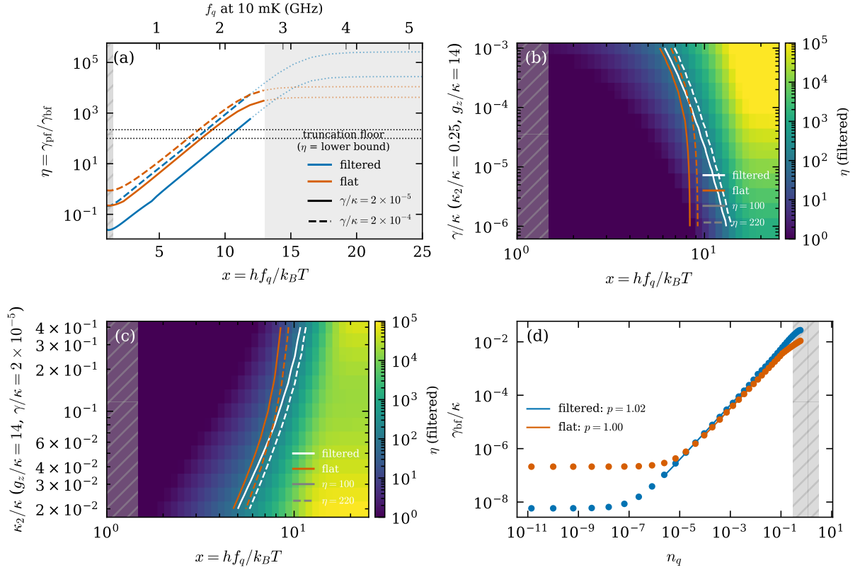
Figura 6: (a) \eta = \gamma_{\text{pf}}/\gamma_{\text{bf}} frente a x = hf_q/k_BT en la región de referencia, con filtro (azul) y baño plano (naranja), para \gamma/\kappa = 2 \times 10^{-5} (continua) y 2 \times 10^{-4} (discontinua). Más allá de x = 13 las curvas (punteadas) son el piso de truncamiento a T \rightarrow 0 y \eta es una cota inferior. (b) Mapa de \eta en (\gamma/\kappa, x) ; (c) en (\kappa_2/\kappa, x) con \gamma/\kappa = 2 \times 10^{-5} . Contornos blancos: baño filtrado; naranjas: plano; continuos \eta = 100 , discontinuos \eta = 220 . (d) \gamma_{\text{bf}}/\kappa frente a n_q , con exponente local p .
