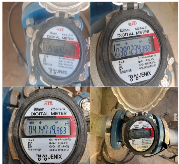
유량계
