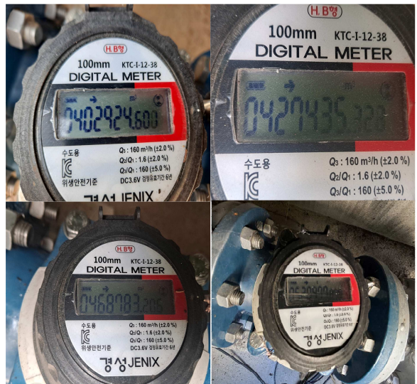
유량계
