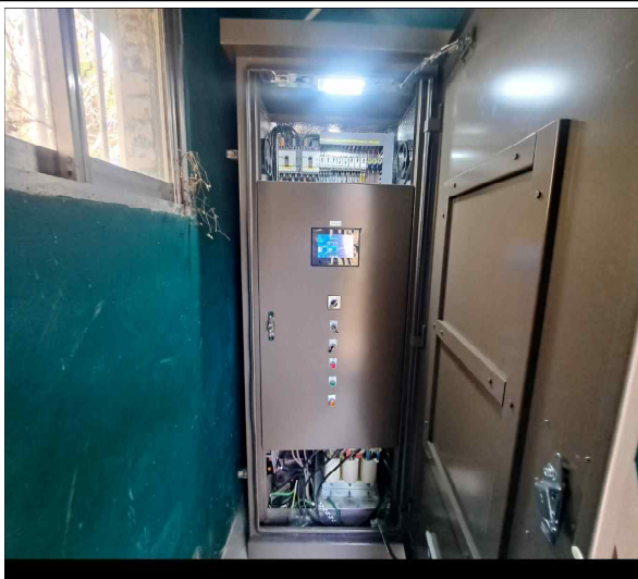
배전반
