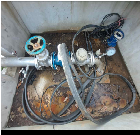
보호시설 내부
