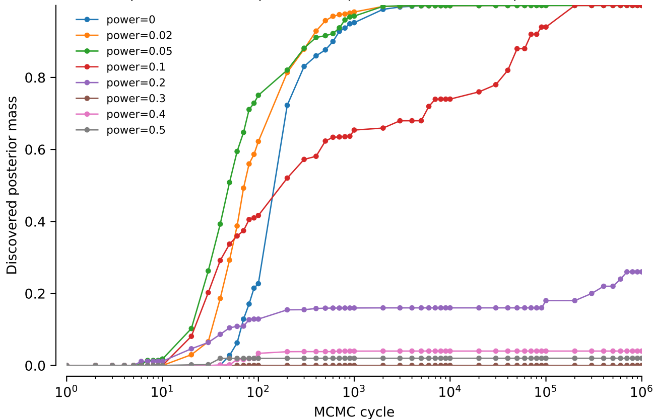
vert.atpase6.tw0: NNI power comparison: Discovered posterior mass
