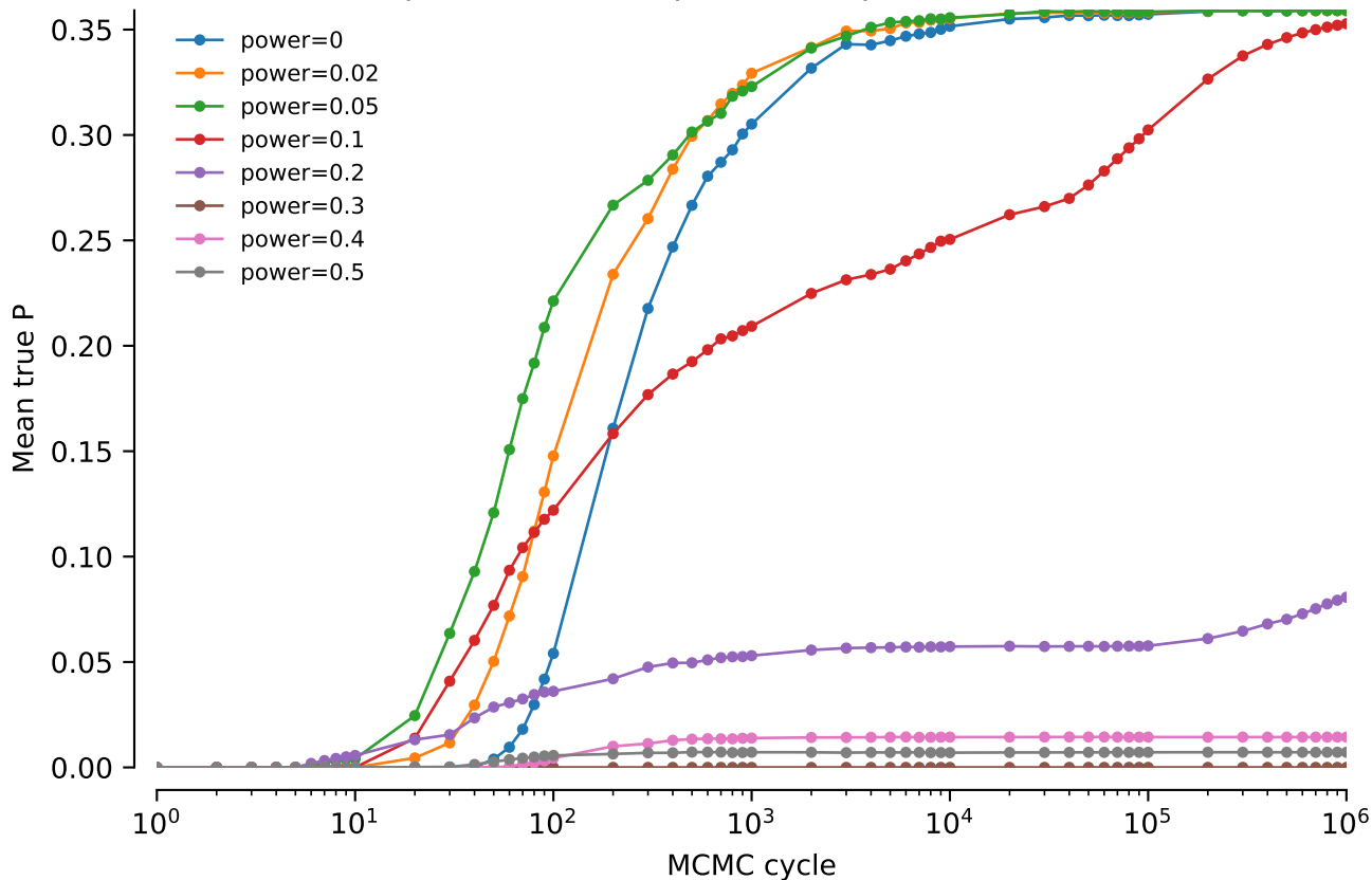
vert.atpase6.tw0: NNI power comparison: Mean true P
