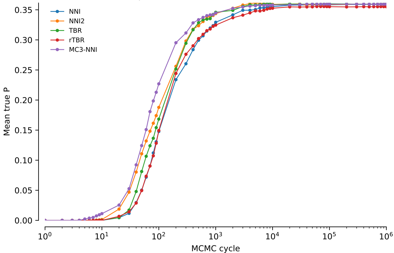
vert.atpase6.tw0: Mean true P: power = 0.02
