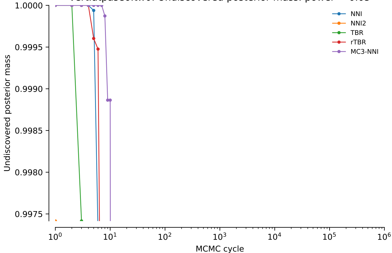
vert.atpase6.tw0: Undiscovered posterior mass: power = 0.05
