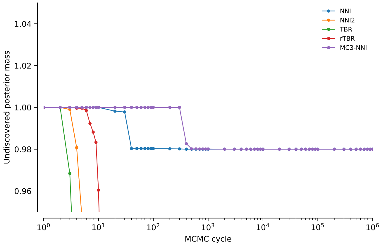
vert.atpase6.tw0: Undiscovered posterior mass: power = 0.5
