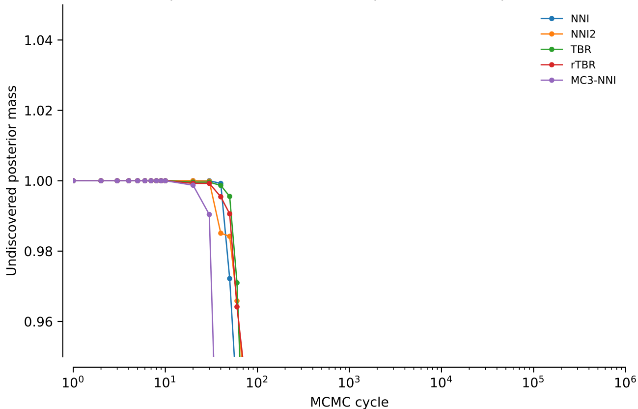
vert.atpase6.tw0: Undiscovered posterior mass: power = 0
