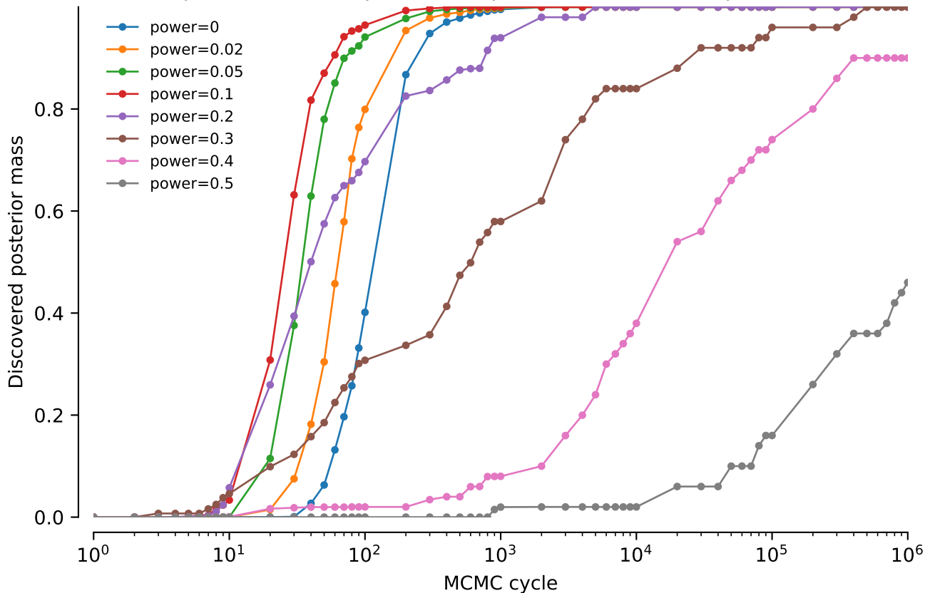
vert.atpase6.tw5: NNI power comparison: Discovered posterior mass
