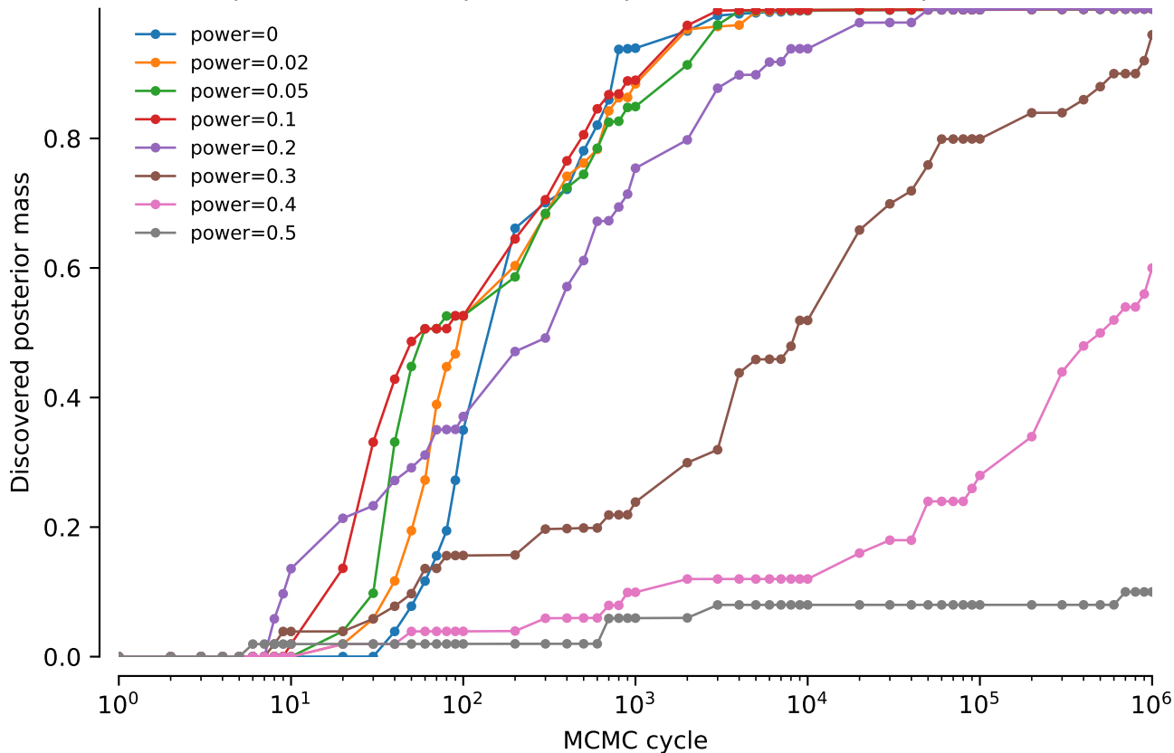
vert.atpase8.tw0: NNI power comparison: Discovered posterior mass
