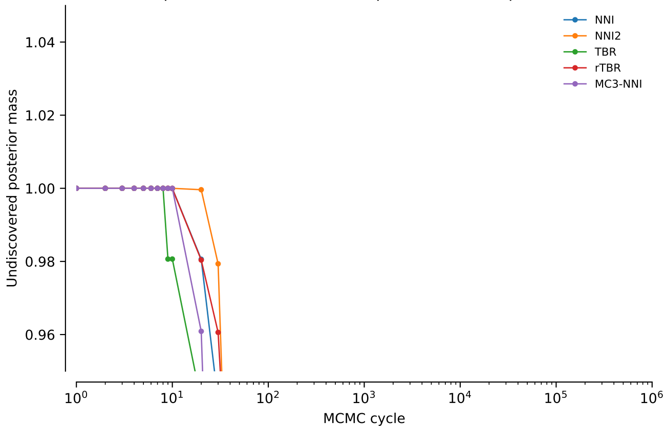
vert.atpase8.tw0: Undiscovered posterior mass: power = 0.02
