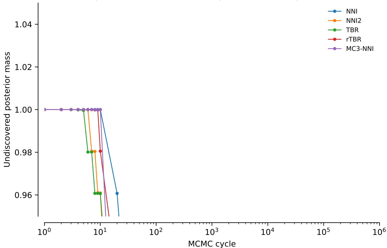
vert.atpase8.tw0: Undiscovered posterior mass: power = 0.05
