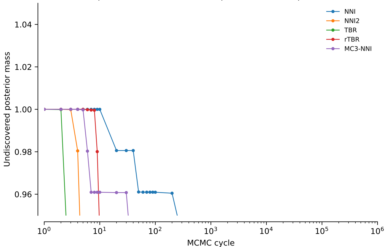
vert.atpase8.tw0: Undiscovered posterior mass: power = 0.4
