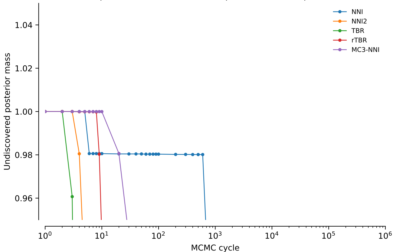
vert.atpase8.tw0: Undiscovered posterior mass: power = 0.5
