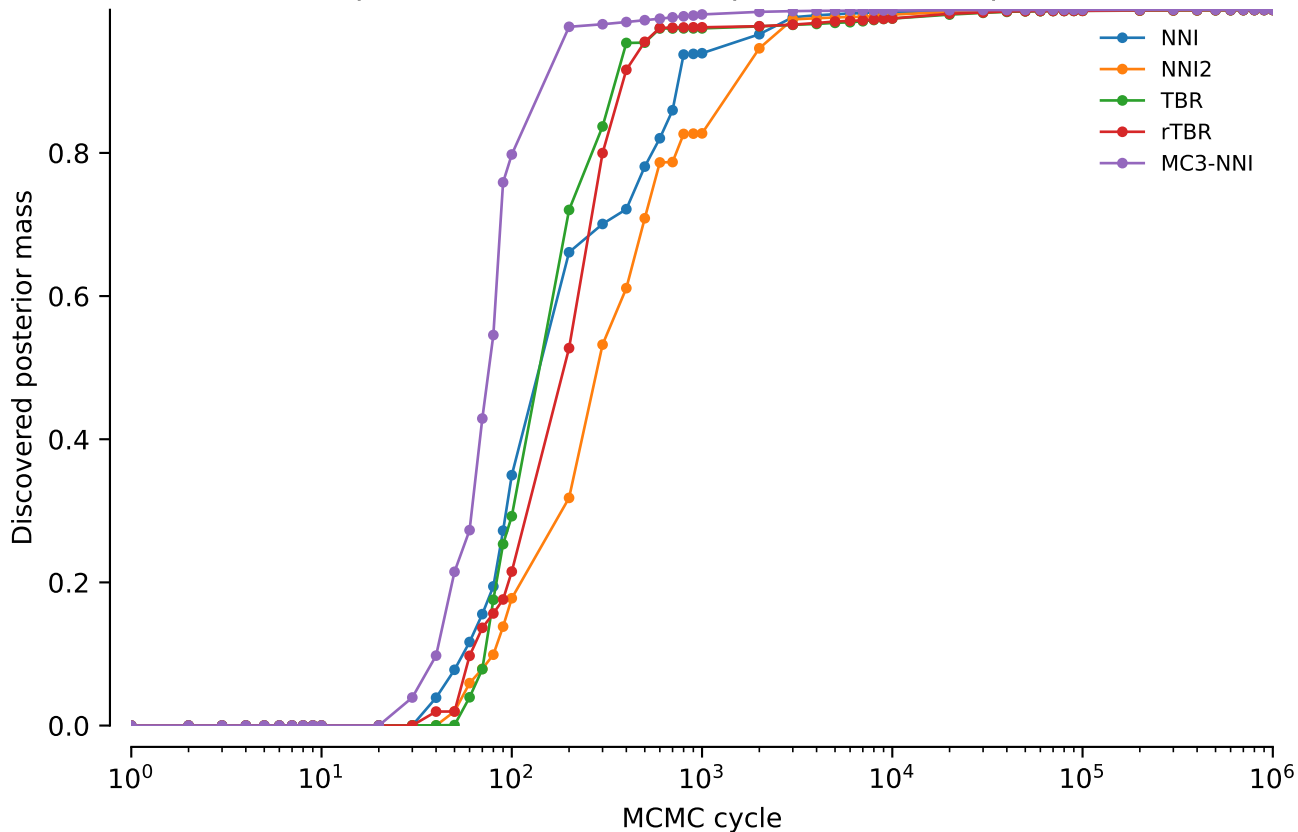
vert.atpase8.tw0: Discovered posterior mass: power = 0
