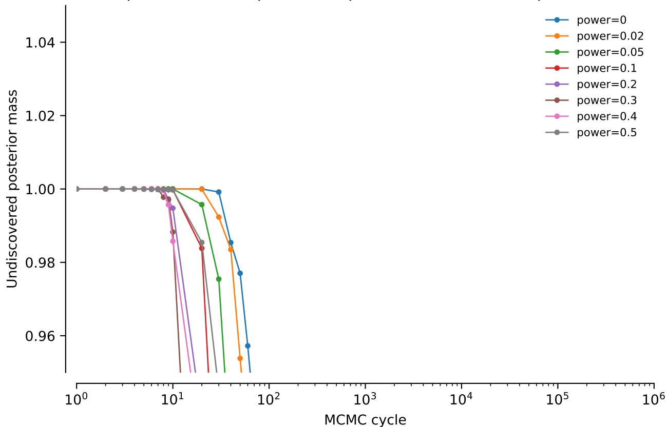
vert.atpase8.tw5: NNI power comparison: Undiscovered posterior mass
