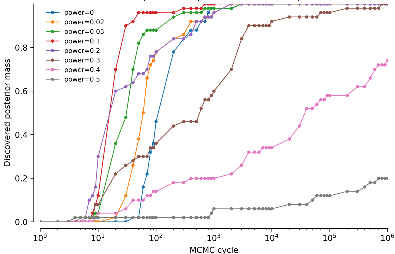
vert.coi.tw0: NNI power comparison: Discovered posterior mass
