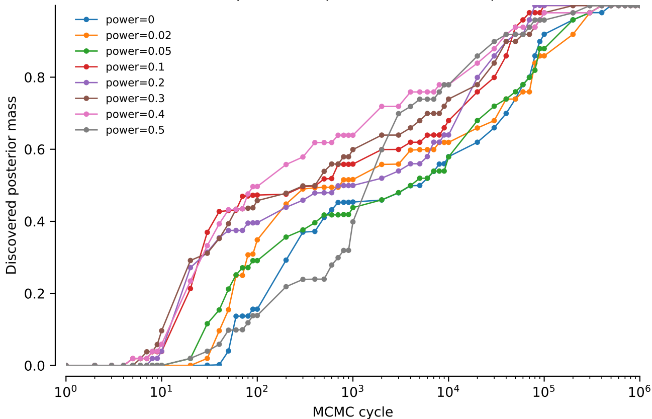
vert.coi.tw5: NNI power comparison: Discovered posterior mass
