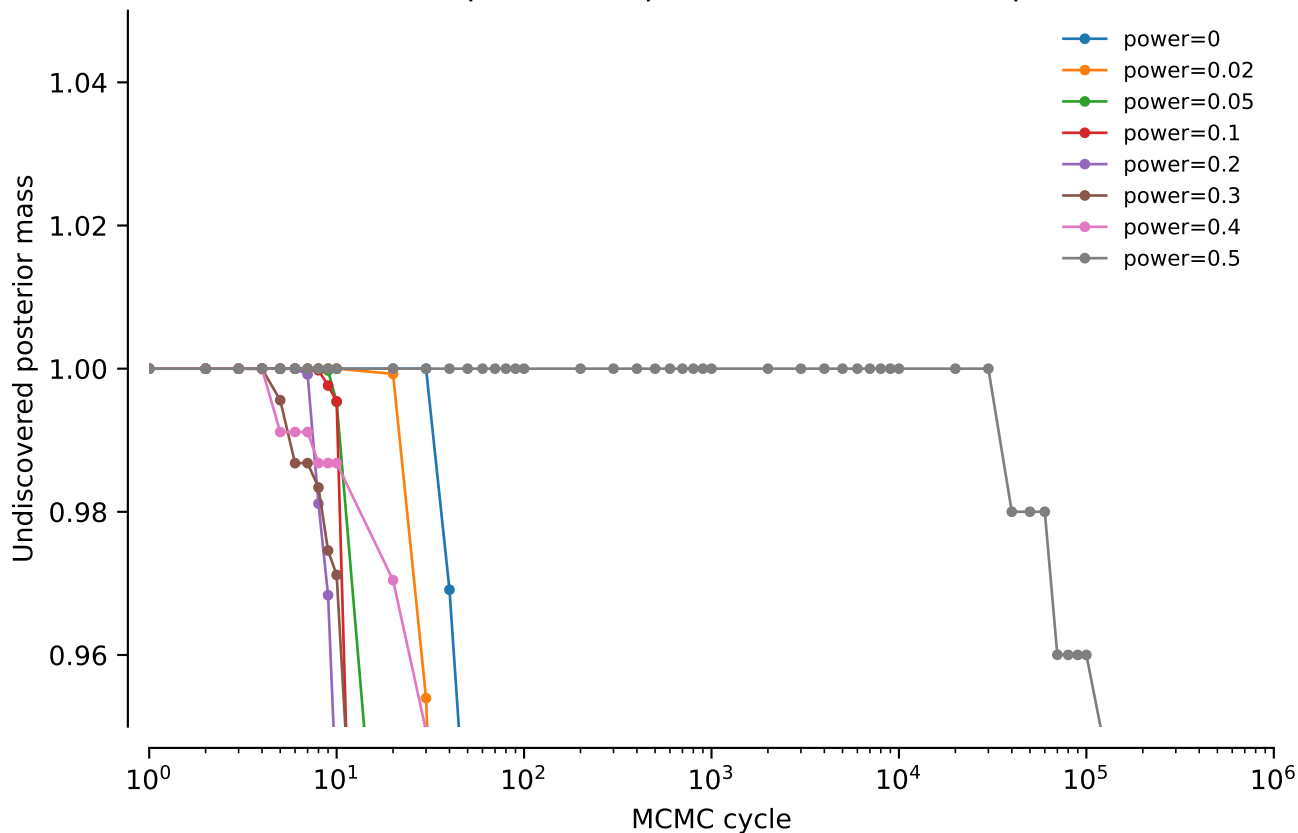
vert.nd3.tw0: NNI power comparison: Undiscovered posterior mass
