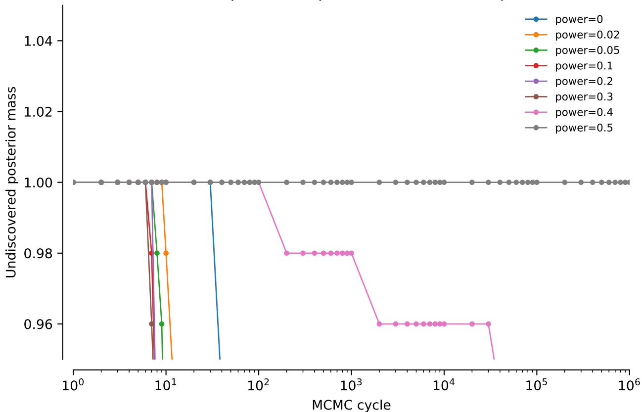
vert.nd4.tw0: NNI power comparison: Undiscovered posterior mass
