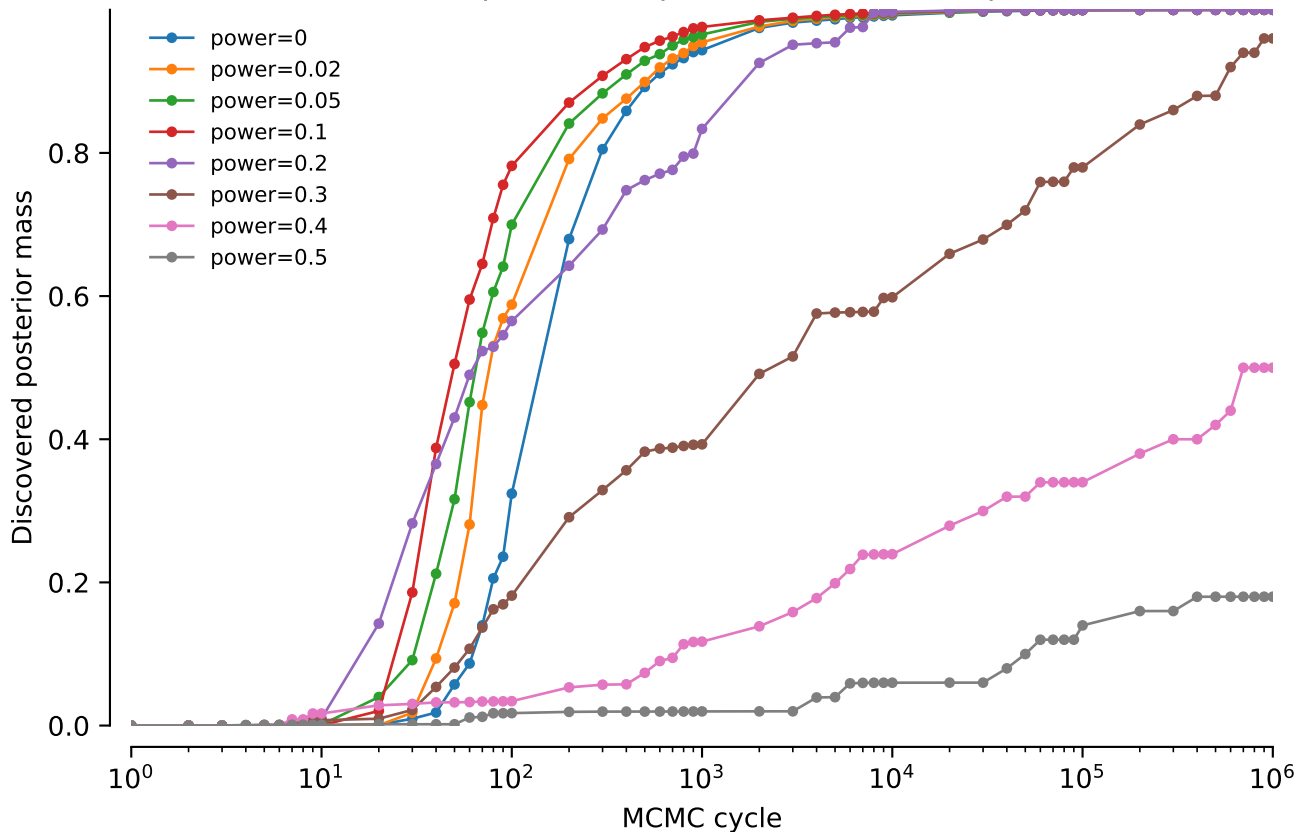
vert.nd4l.tw0: NNI power comparison: Discovered posterior mass
