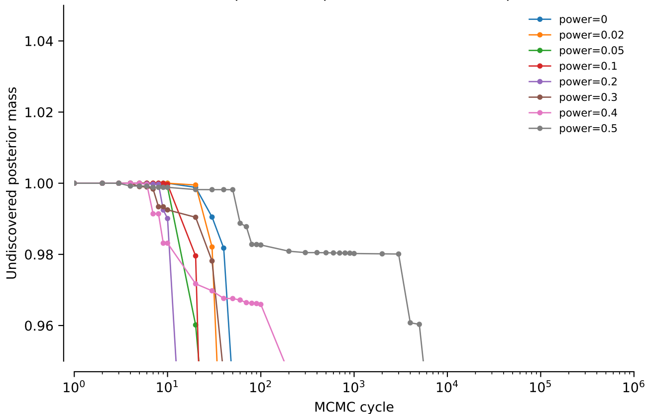
vert.nd4l.tw0: NNI power comparison: Undiscovered posterior mass
