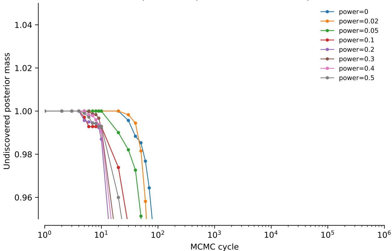
vert.nd4l.tw5: NNI power comparison: Undiscovered posterior mass
