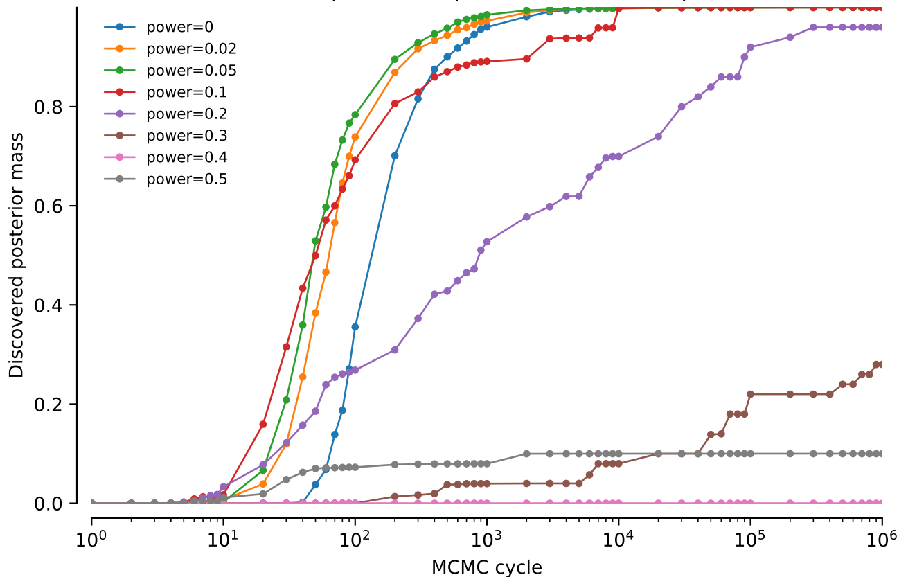
vert.nd6.tw0: NNI power comparison: Discovered posterior mass
