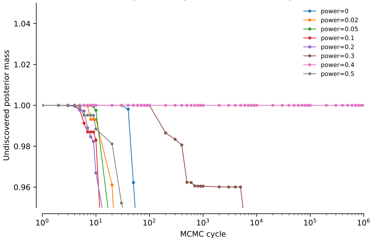
vert.nd6.tw0: NNI power comparison: Undiscovered posterior mass
