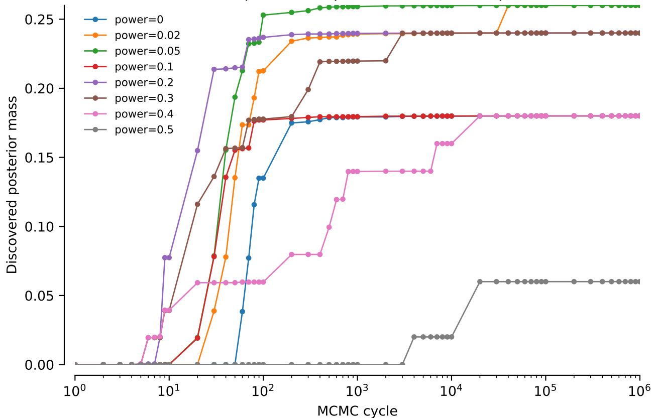
vert.nd6.tw5: NNI power comparison: Discovered posterior mass
