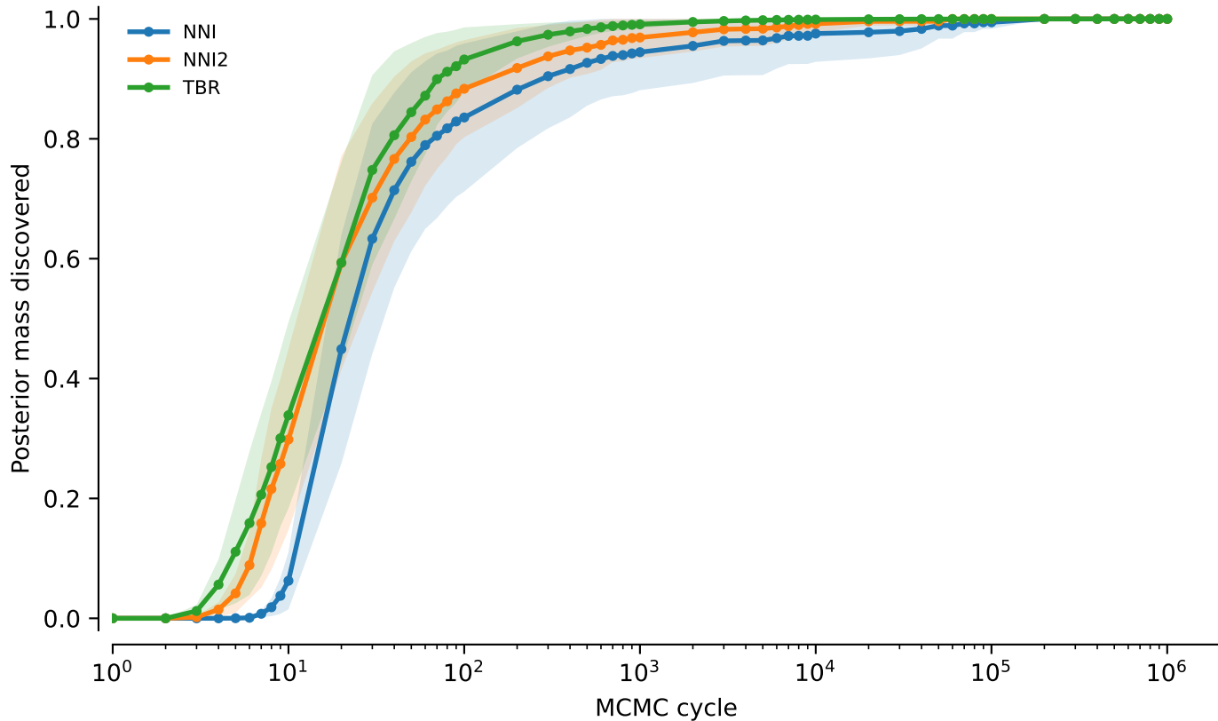
tw0: NNI vs NNI2 vs TBR, power=0.1: Posterior mass discovered
