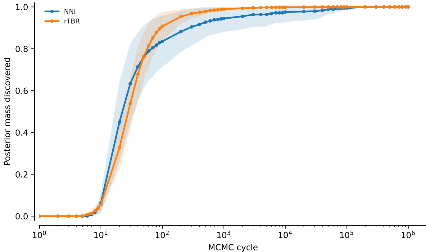
tw0: NNI vs rTBR, power=0.1: Posterior mass discovered
