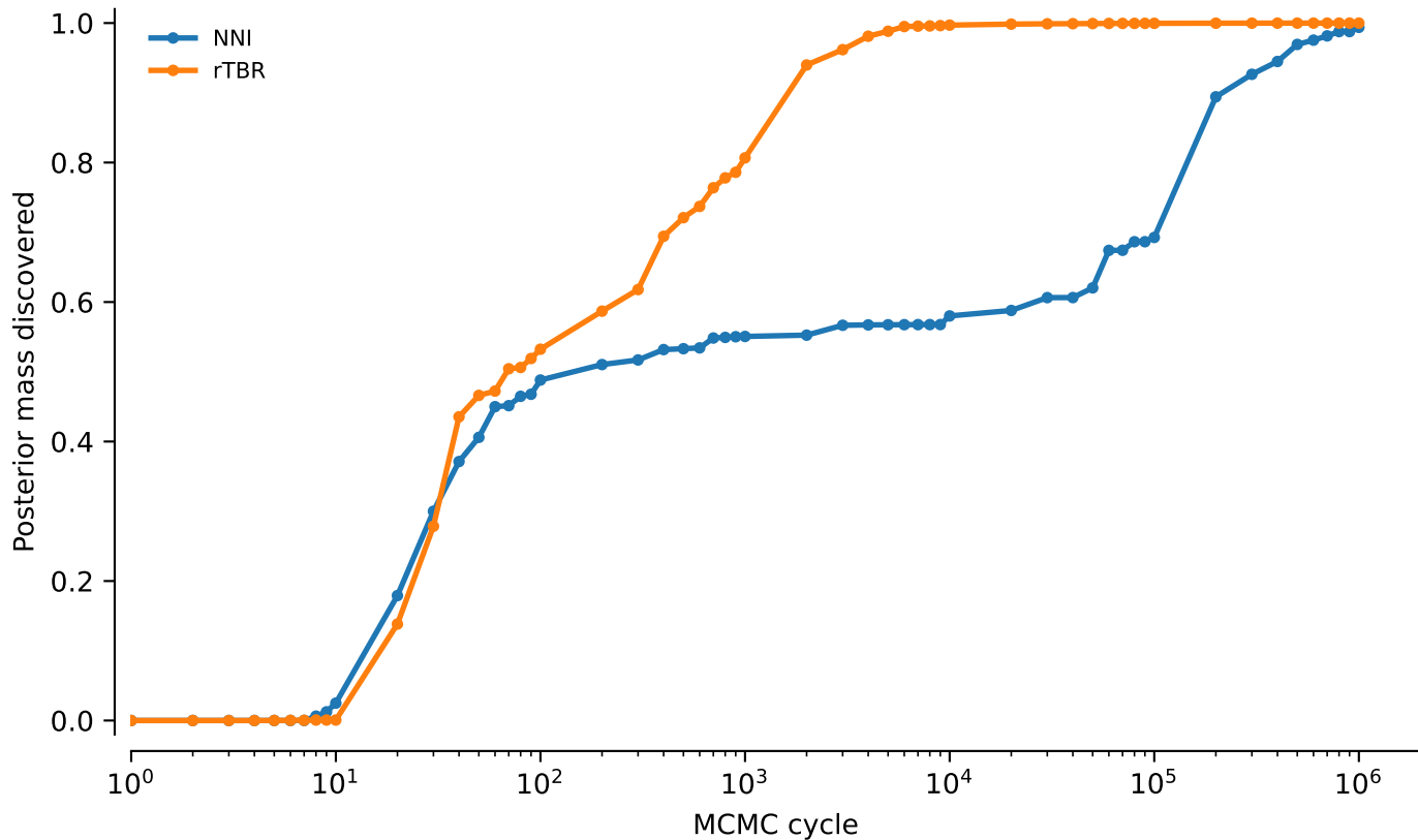
tw2: NNI vs rTBR, power=0.1: Posterior mass discovered
