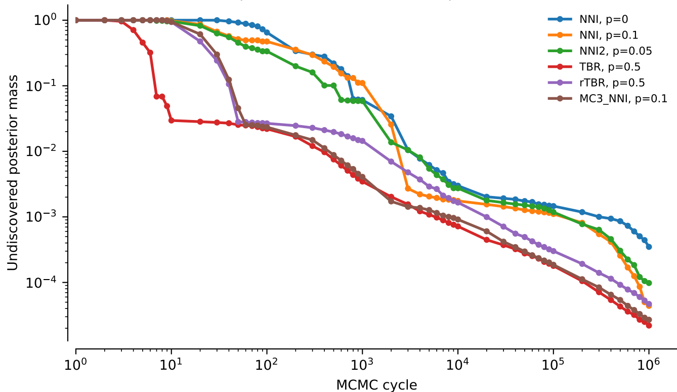
vert.atpase8.tw0: undiscovered posterior mass
