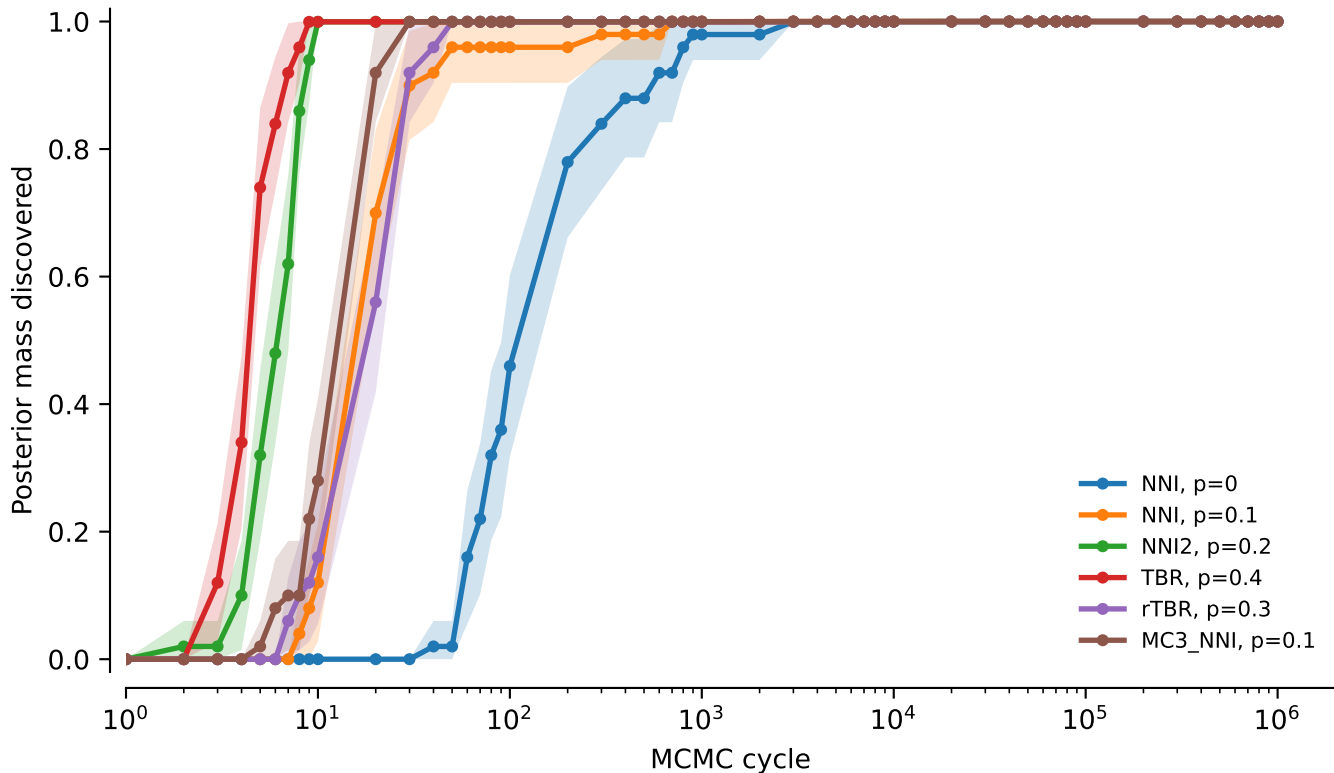
vert.coi.tw0: Posterior mass discovered
