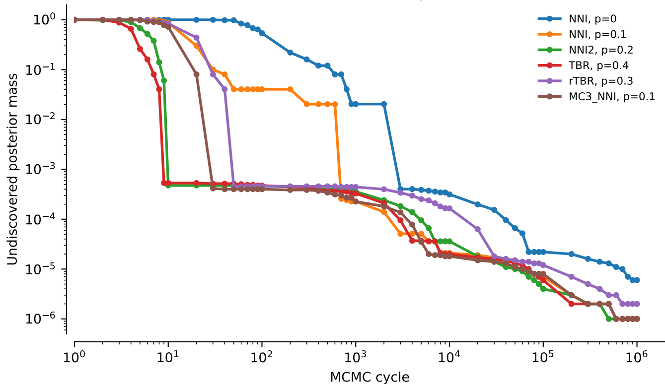
vert.coi.tw0: undiscovered posterior mass
