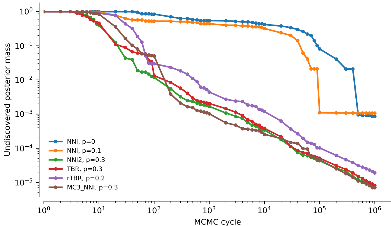
vert.coi.tw5: undiscovered posterior mass
