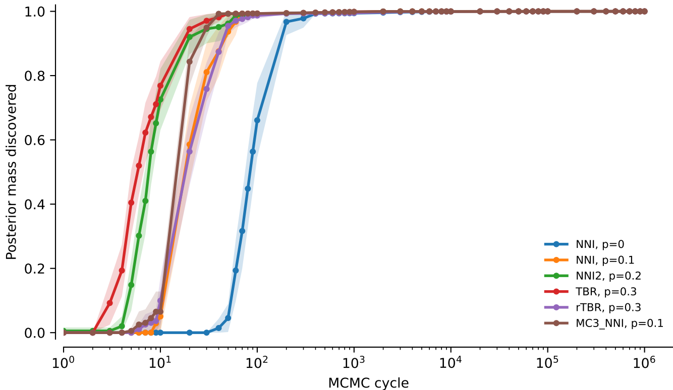
vert.coii.tw0: Posterior mass discovered
